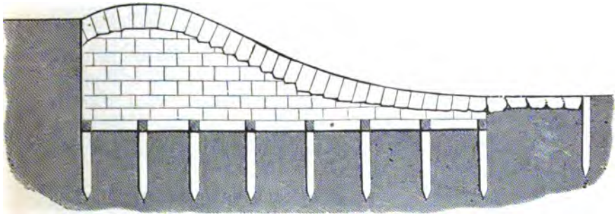
Fig. 246.—Stone weir.
